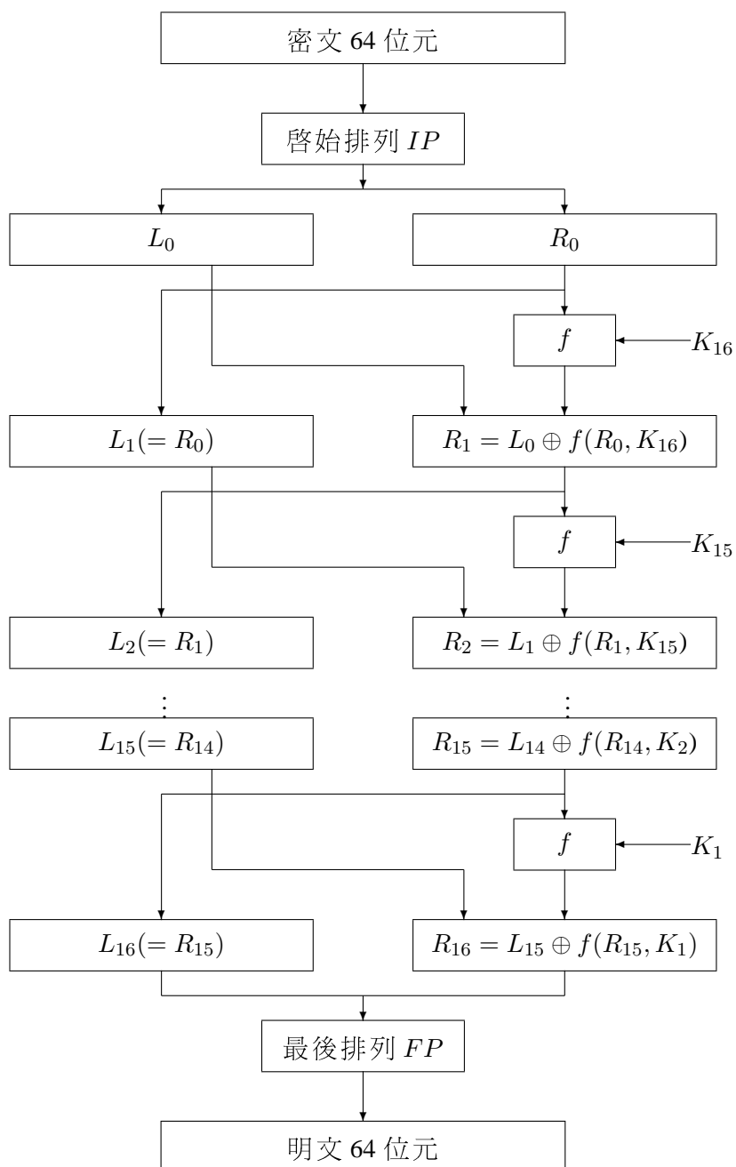
圖 5.6: DES 解密過程
